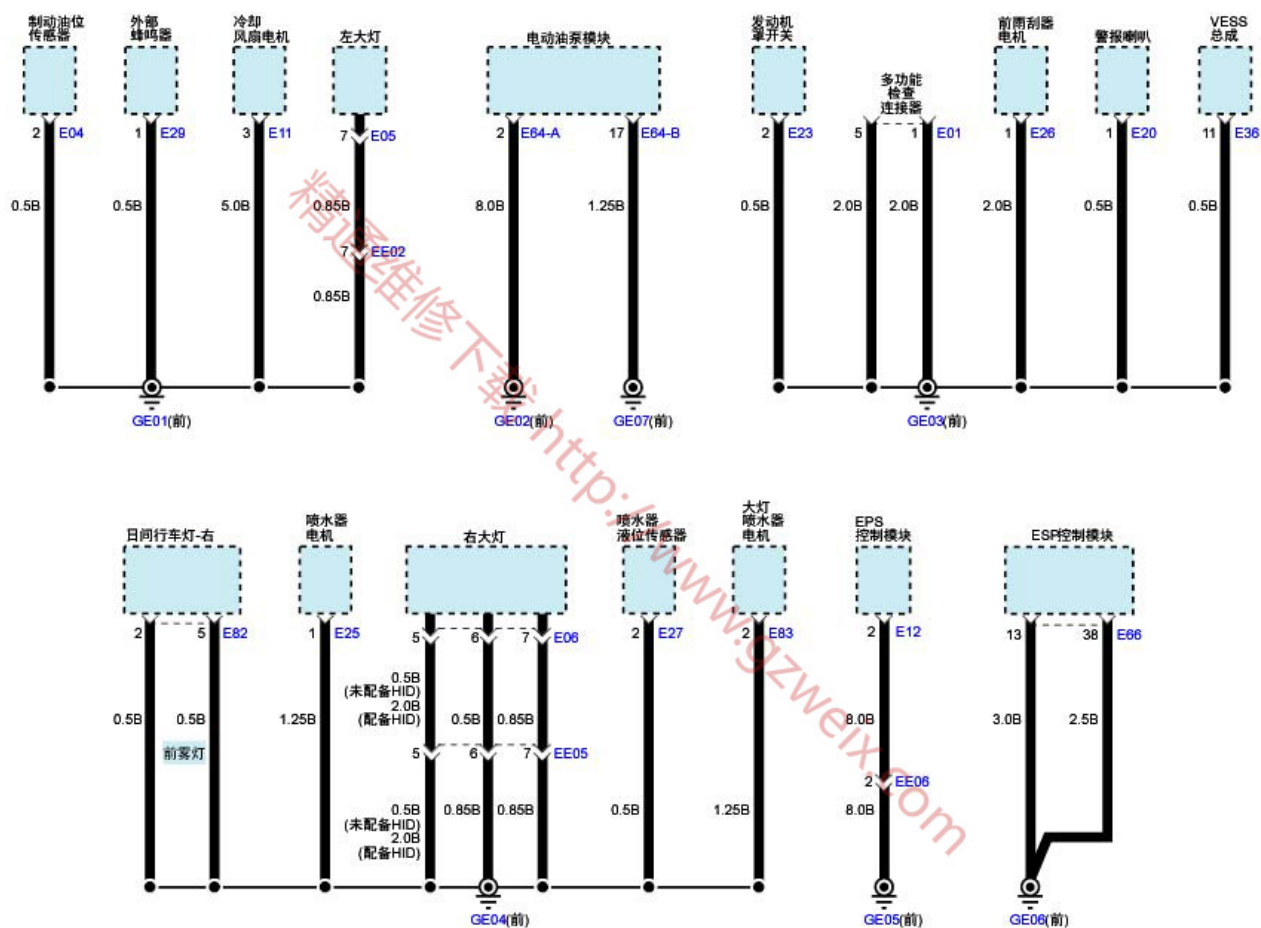
搭铁分布(3)
